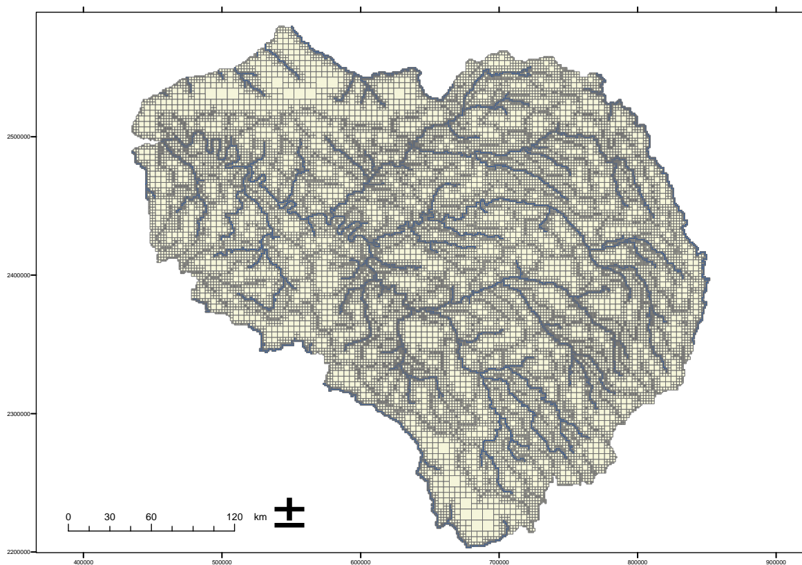
Figure 11 : réseau hydrographique « modèle »
