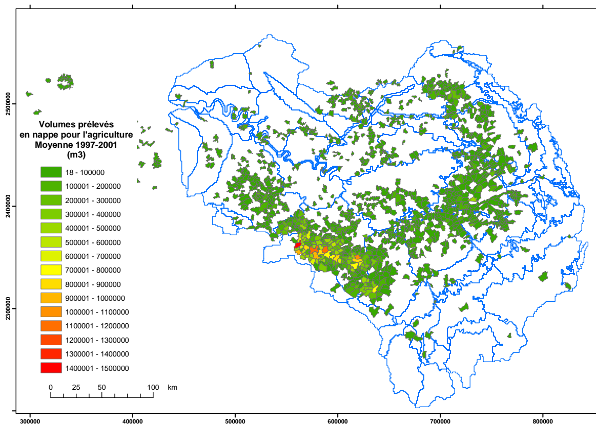
Figure 1 : moyenne des prélèvements agricoles agrégés par commune (moyenne des années 1997-2001)
