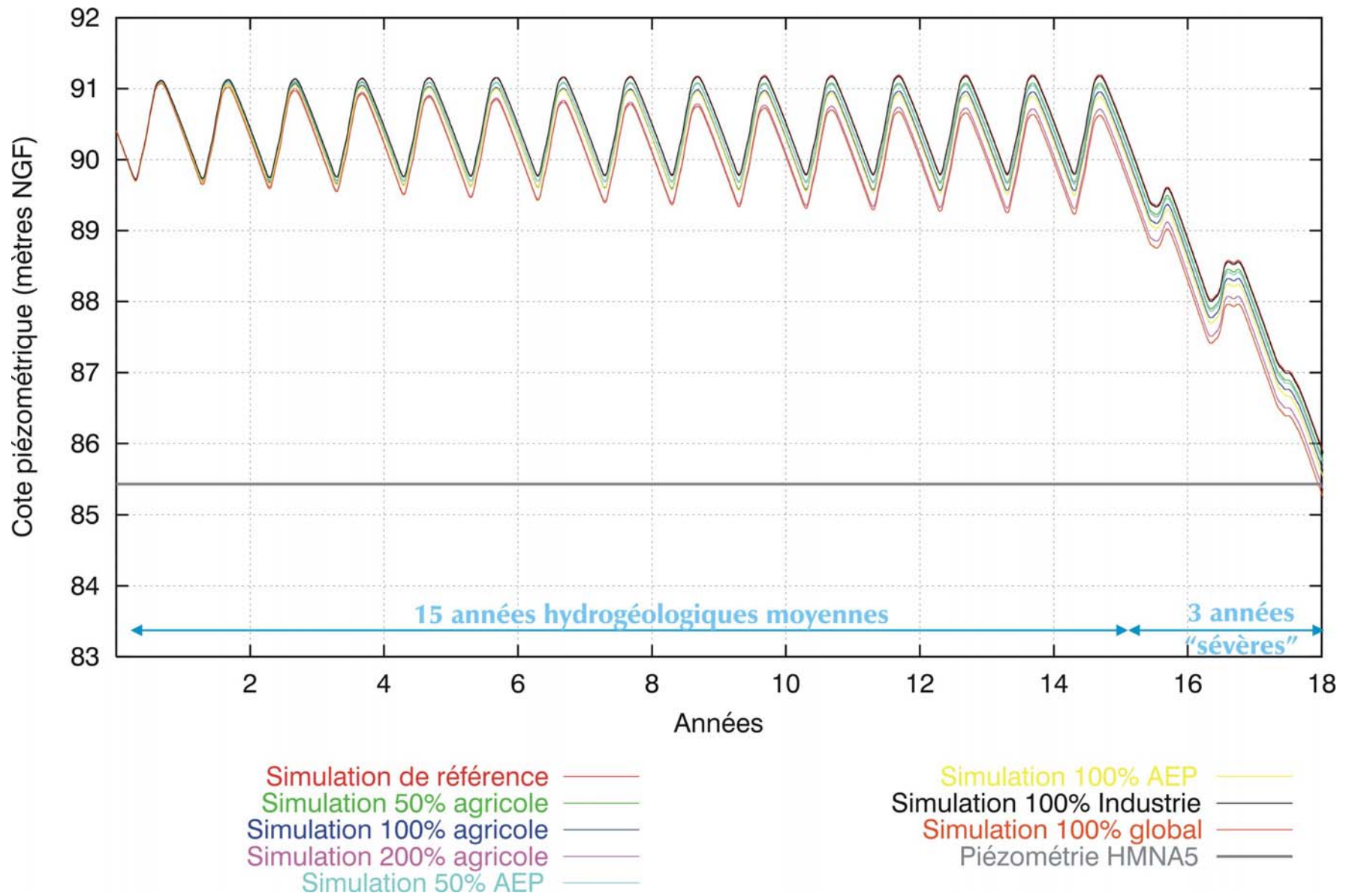
Figure 84 : évolution piézométrique calculée au piézomètre de Lagny - formation Eocène
