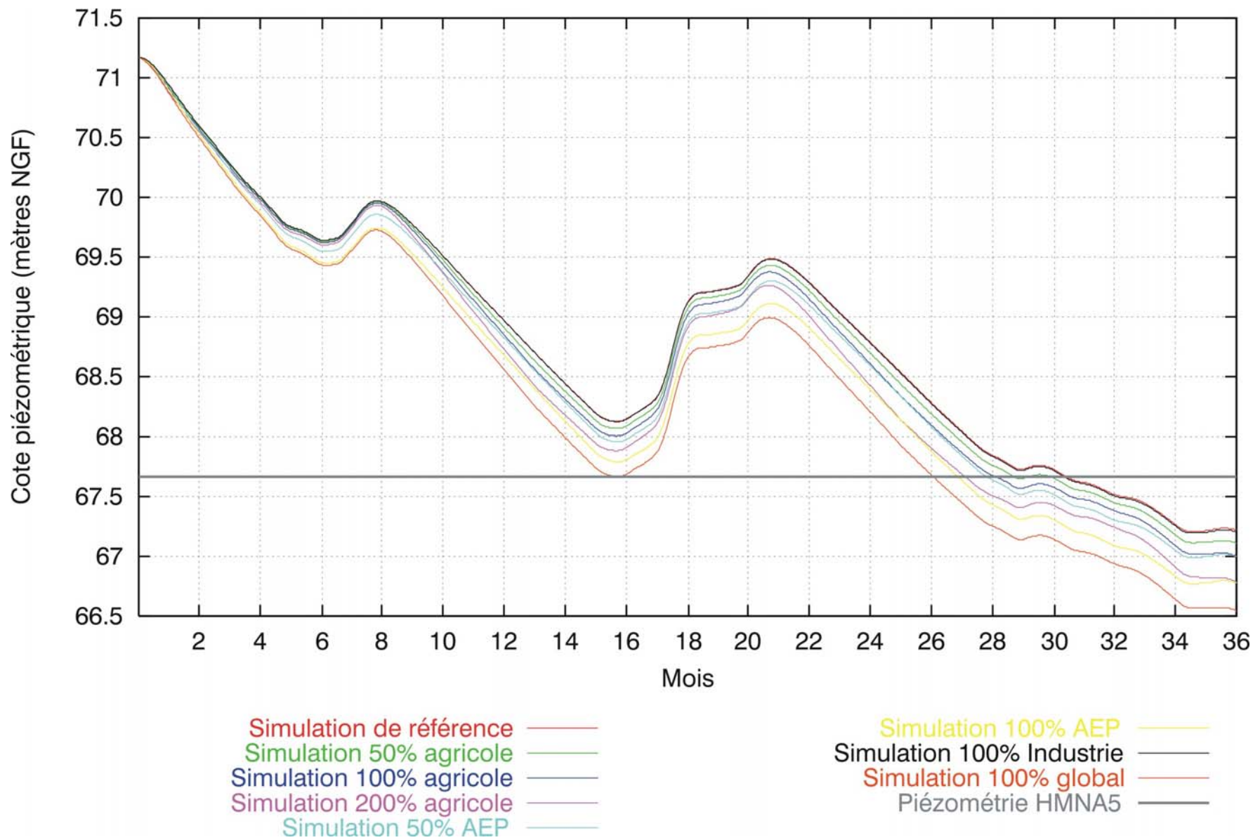
Figure 100 : évolution piézométrique calculée sur trois années climatiques « sévères » au piézomètre de Laon - formation de la Craie
