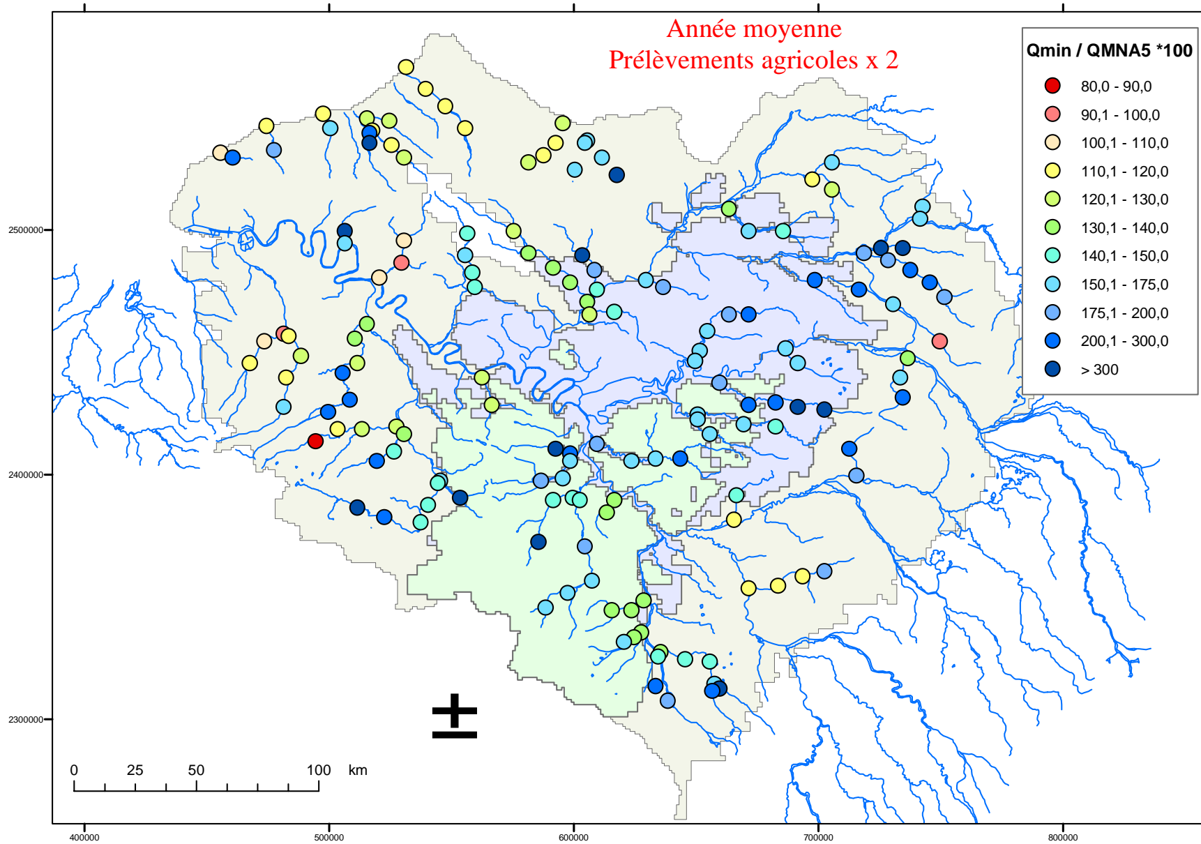
Figure 52 : rapport Q_{min} moyen mensuel / QMNA5 calculé en année moyenne avec doublement des prélèvements agricoles
