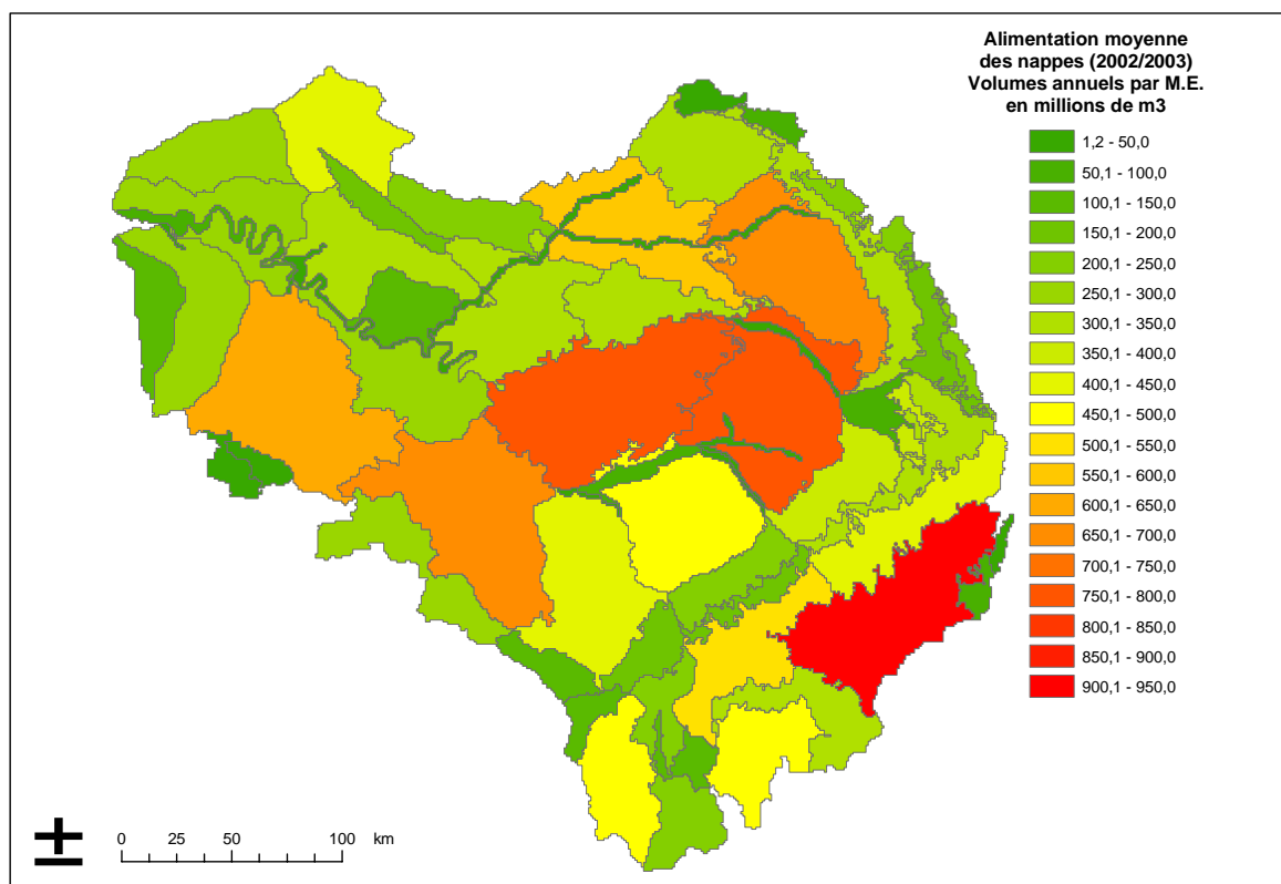
Figure 20 : alimentation efficace moyenne des nappes rapportée aux masses d'eau de la DCE
