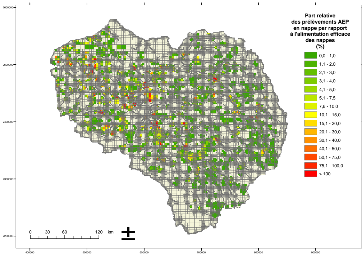
Figure 24 : part relative prélèvements AEP / alimentation des nappes
