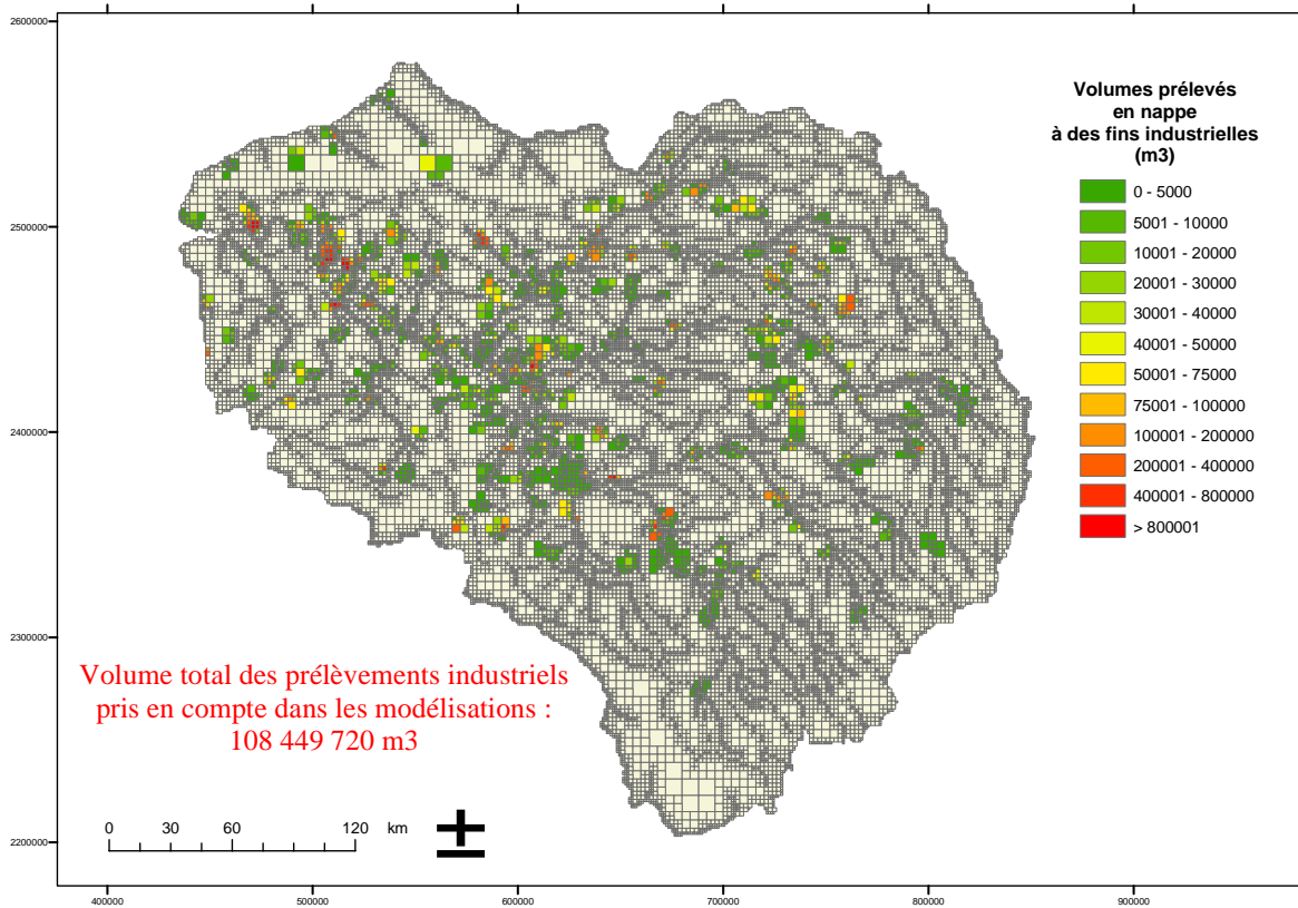
Figure 15 : prélèvements industriels 2004 en nappes rapportés au maillage de surface du modèle
