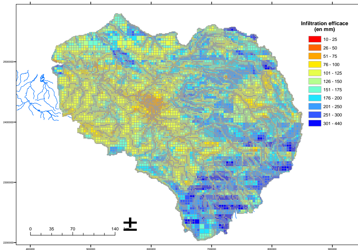
Figure 19 : infiltration moyenne calculée – année 2002-2003
