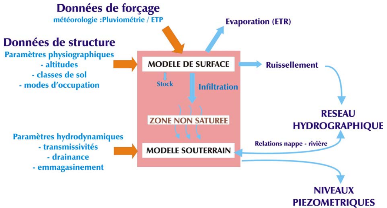
Figure 4 : principe général du modèle hydrogéologique couplé MODCOU
