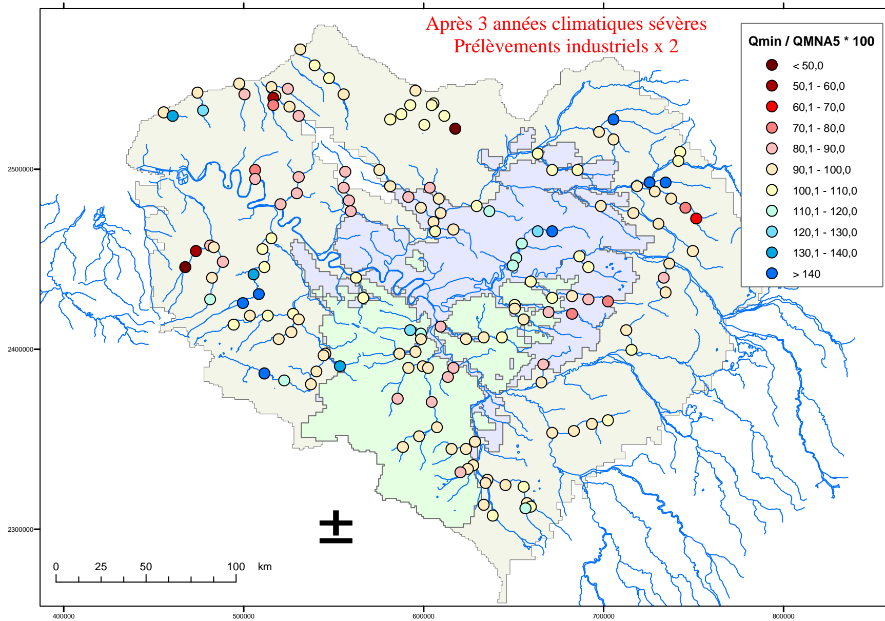
Figure 64 : rapport Q_{min} moyen mensuel / QMNA5 calculé après trois années « sévères » avec doublement des prélèvements industriels
