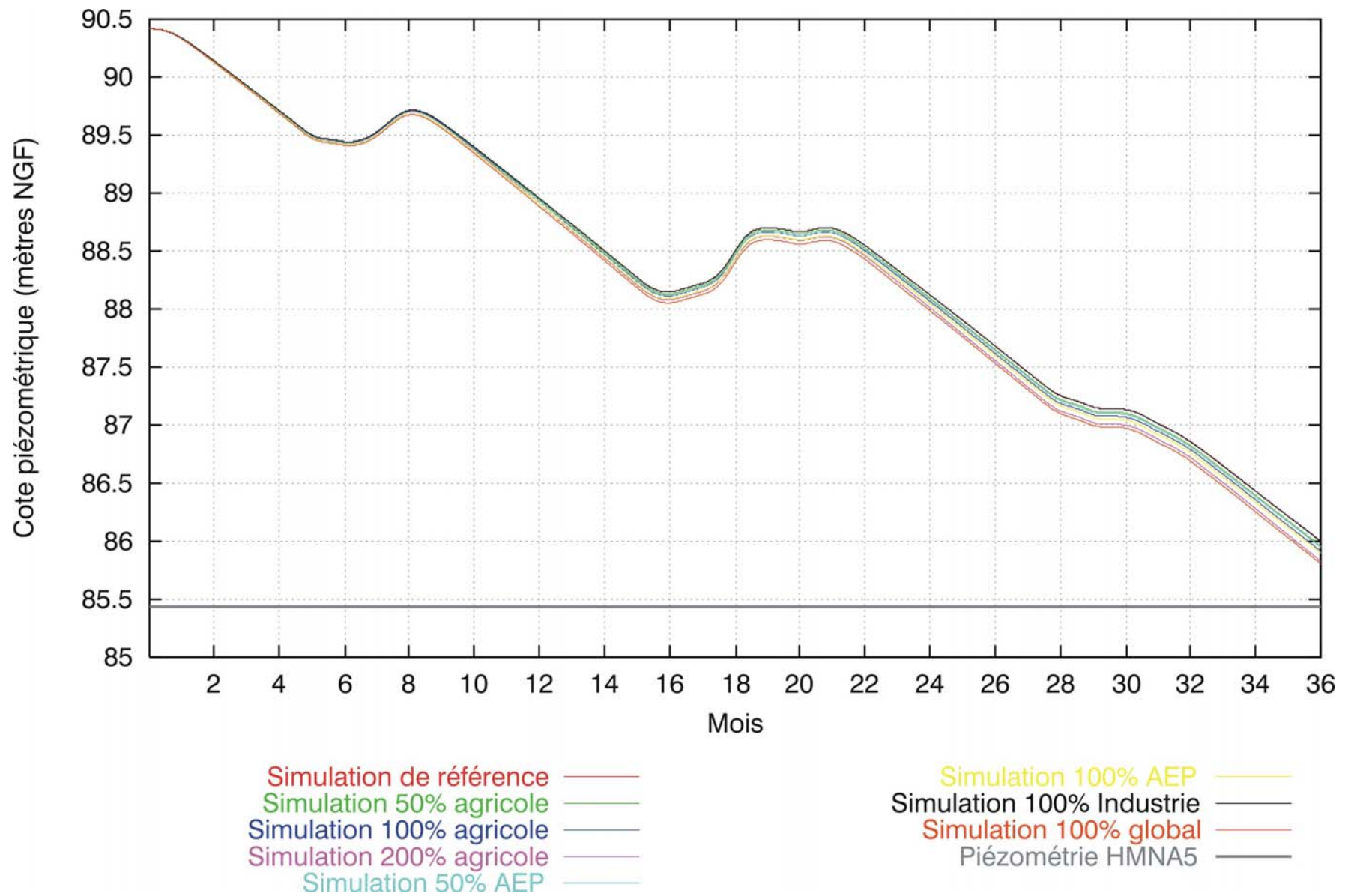
Figure 96 : évolution piézométrique calculée sur trois années climatiques « sévères » au piézomètre de Lagny - formation de l'Eocène
