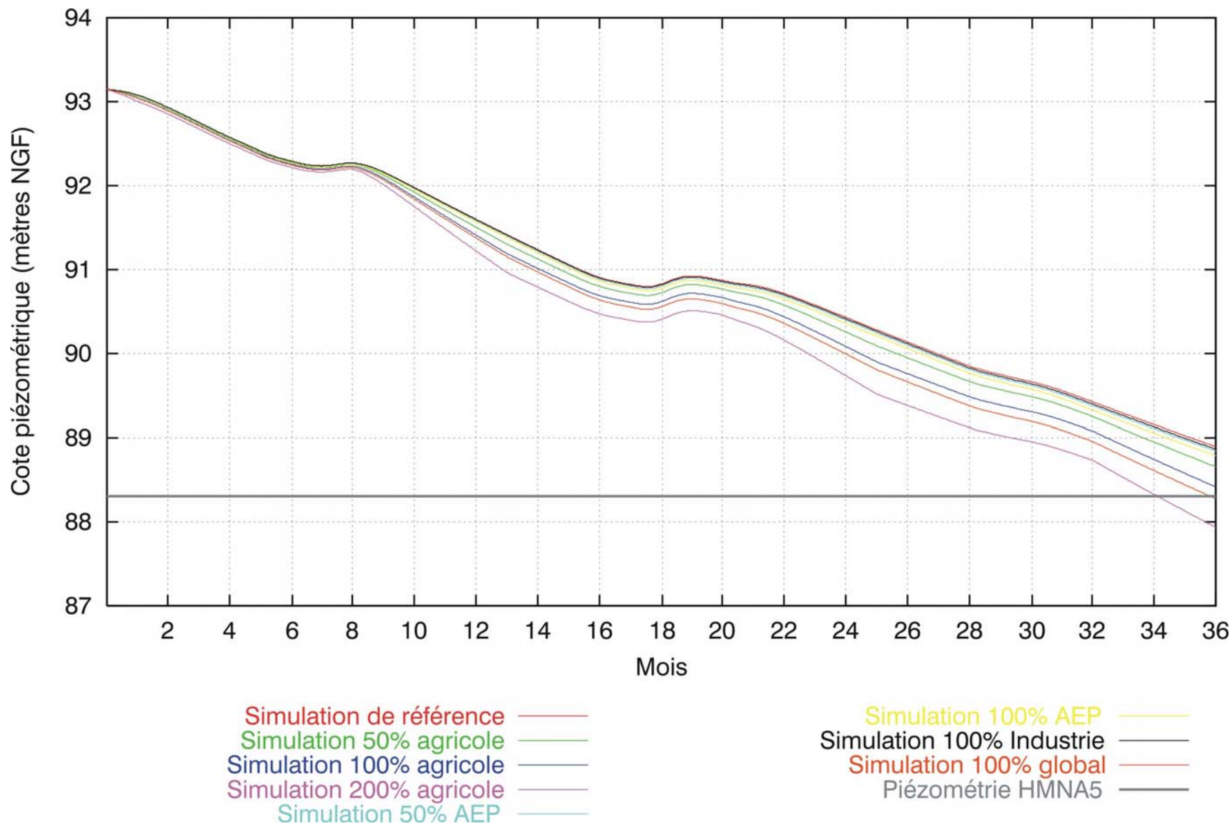
Figure 93 : évolution piézométrique calculée sur trois années climatiques « sévères » au piézomètre de Mainvilliers - formation de l'Oligocène
