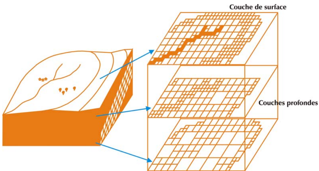
Figure 5 : principe de la schématisation multicouche
