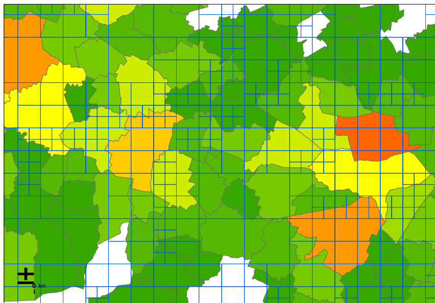
Figure 10 : croisement communes – mailles du modèle de surface
