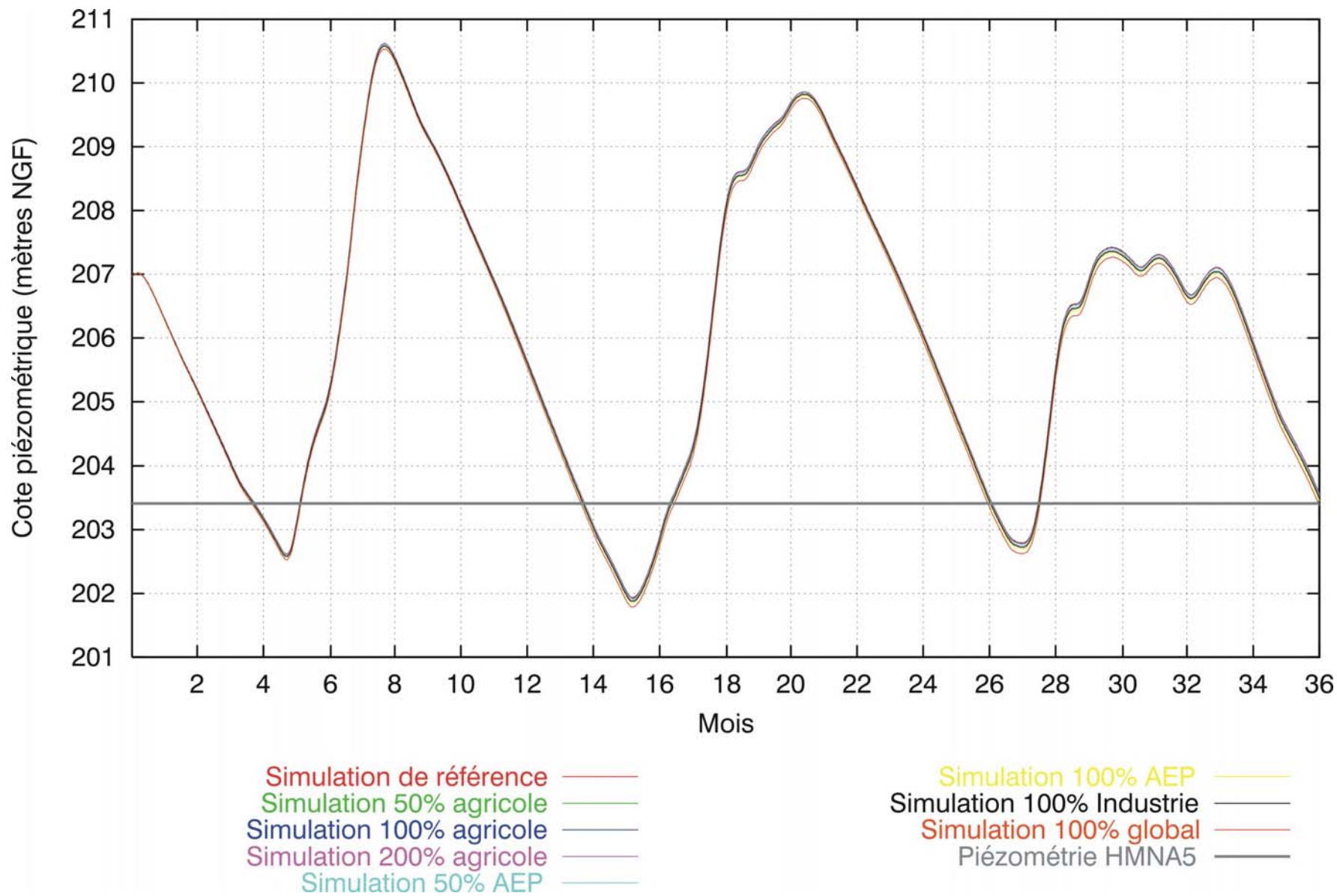
Figure 102 : évolution piézométrique calculée sur trois années climatiques « sévères » au piézomètre d'Aigles - formation de la Craie
