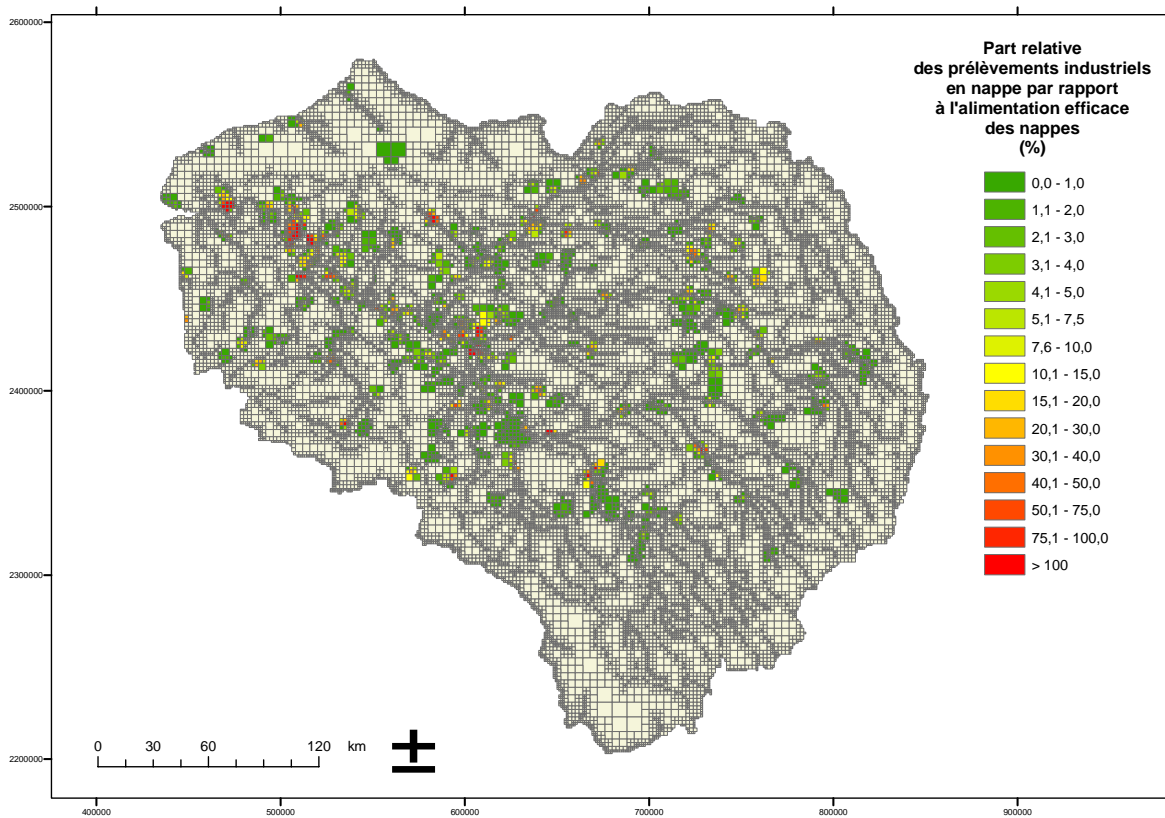
Figure 23 : part relative prélèvements industriels / alimentation des nappes
