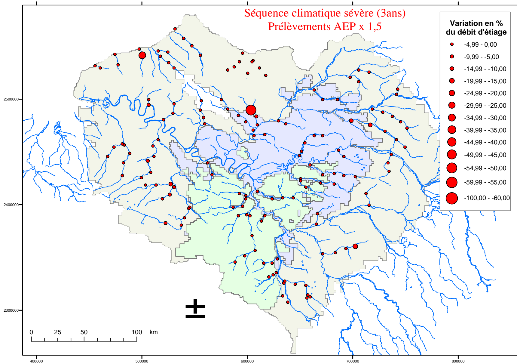
Figure 46 : variations relatives calculées du débit d'été en période climatique sévère liées à une augmentation de 50% des prélèvements AEP
