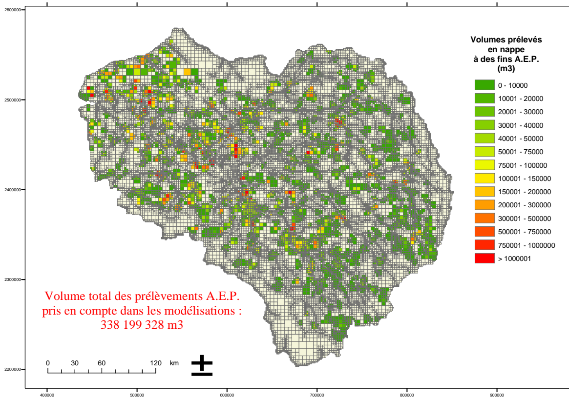
Figure 14 : prélèvements AEP 2004 en nappes rapportés sur le maillage de surface du modèle
