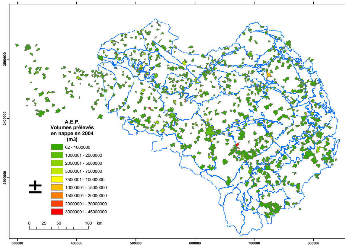
Figure 3 : volumes prélevés en nappe pour l'AEP en m 3 /an : année 2004
