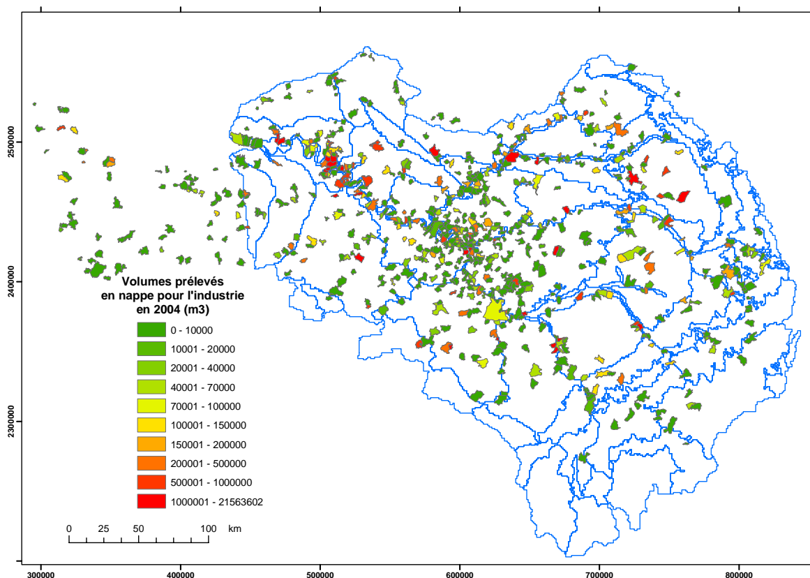
Figure 2 : volumes prélevés en nappe à des fins industrielles en m^3 /an : année 2004
